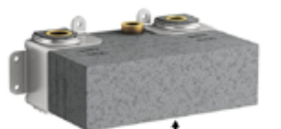
Un boîtier à encastrer ultra-compact Profondeur d'encastrement entre 80 et 100 mm
