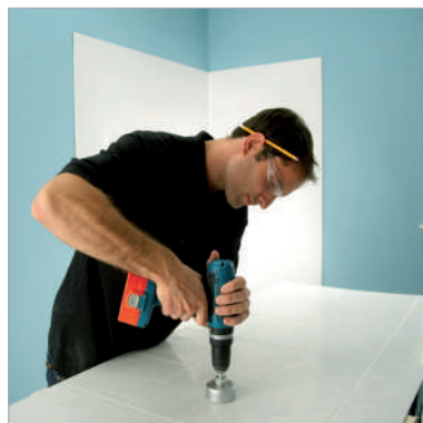
2. Perçage des arrivées d'eau
