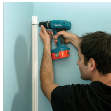
3. Vissage de la cornière d'angle
